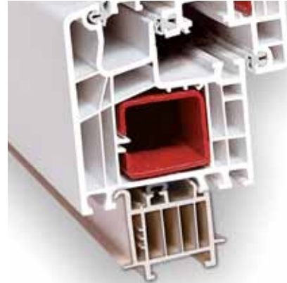
5-komorový osadzovací profil s gumeným tesnením, ktorý znižuje tepelné straty v pripojení okna na parapetné murivo.
