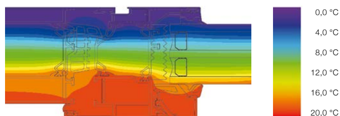
Lineární průběh teplotních izoterm v okně W 77HI zaručuje konstantní průběh teploty podél celého profilu.
